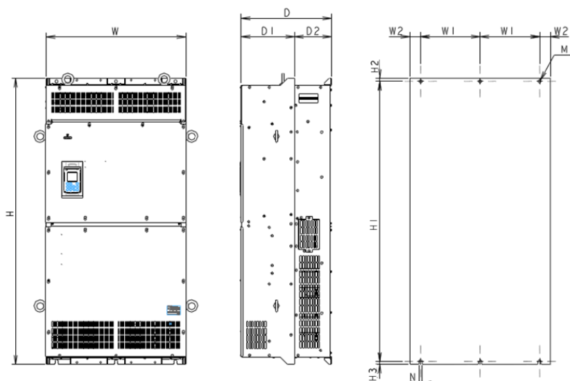
Figura 4 Dimensioni d'ingombro dell'inverter (FRN220AR1S-4□ a FRN400AR1S-4□)
