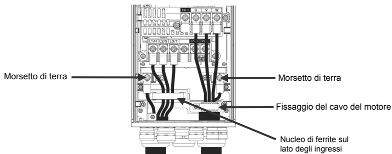
Figura 8.1 Cablaggio dei morsetti del circuito principale per gli inverter di potenza compresa tra 30 e 37 kW
