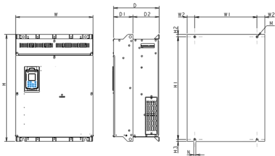
Figura 3 Dimensioni d'ingombro dell'inverter (FRN110AR1S-4□ a FRN200AR1S-4□)
