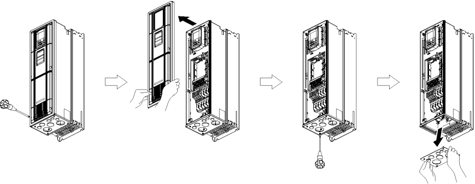
Figura 2.2 Rimozione del coperchio anteriore e della piastra di cablaggio (FRN37AR1M-4□)
