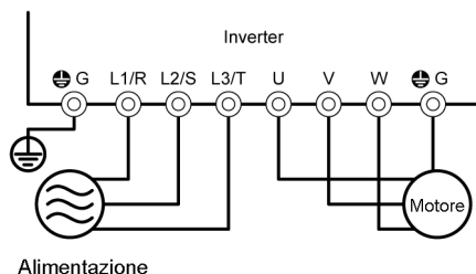
Figura 4.1 Collegamento dei morsetti del circuito principale
