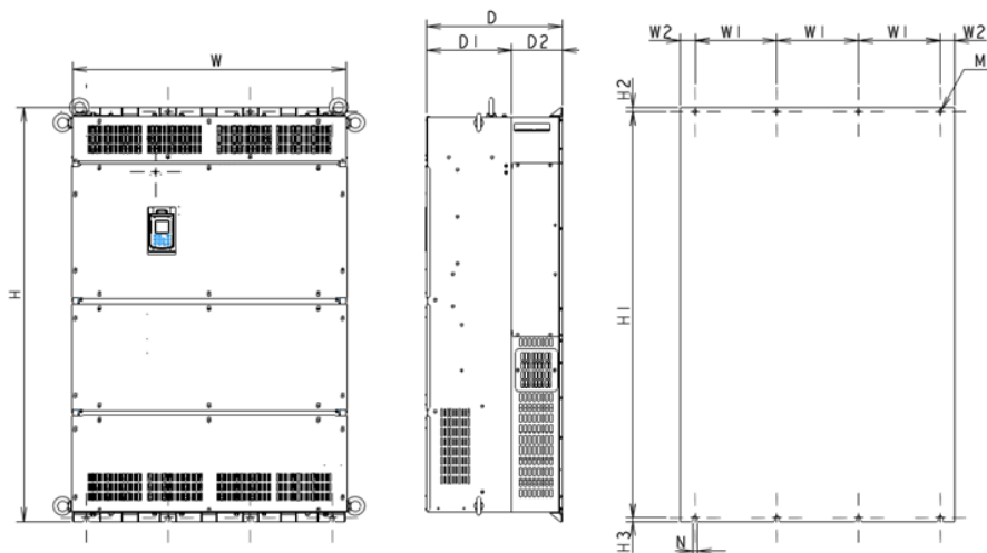
Figura 5 Dimensioni d'ingombro dell'inverter (FRN500AR1S-4□ a FRN710AR1S-4□)
