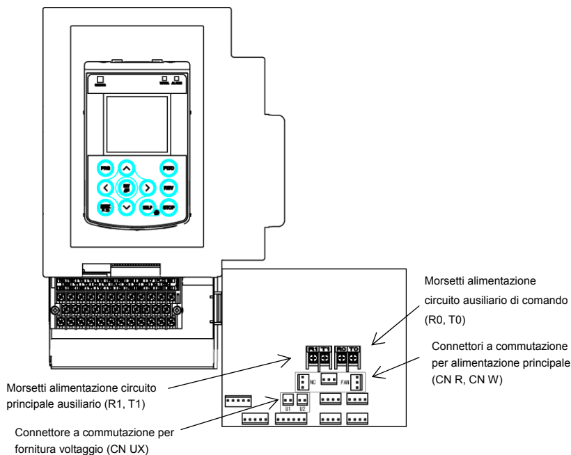
Figura 2.7 Posizione dei connettori a commutazione (160 kW o più)
