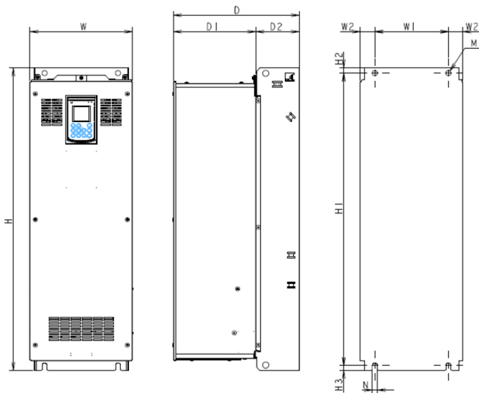
Figura 2 Dimensioni d'ingombro dell'inverter (FRN45AR1■-4□ a FRN90AR1■-4□)
