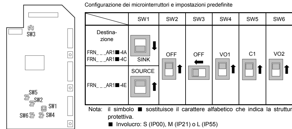
Figura 2.9 Posizione dei microinterruttori a slitta sulla scheda di comando a circuito stampato
