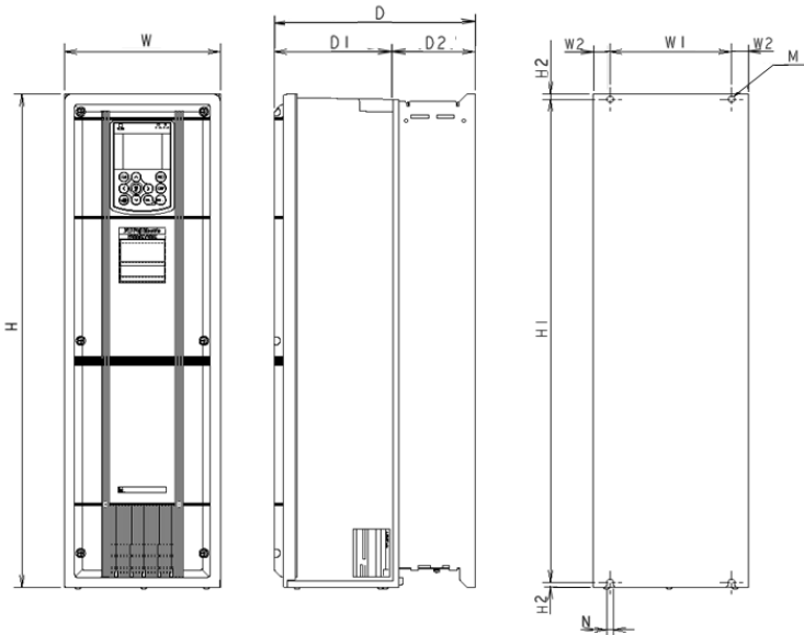
Figura 1 Dimensioni d'ingombro dell'inverter (FRN0.75AR1■-4□ a FRN37AR1■-4□)
