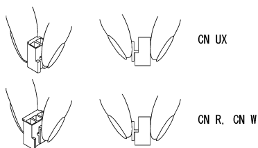
Figura 2.8 Inserimento o rimozione di un connettore a commutazione (45 kW o più)
